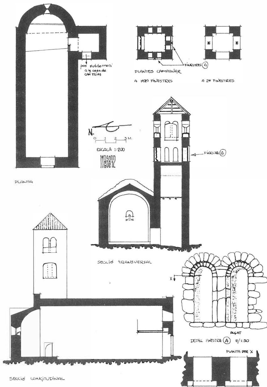
Santa Maria de Toudell. (Planimetria: J. M. Masagué.)
